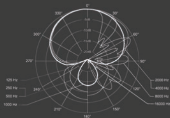
强指向性拾音示意图
